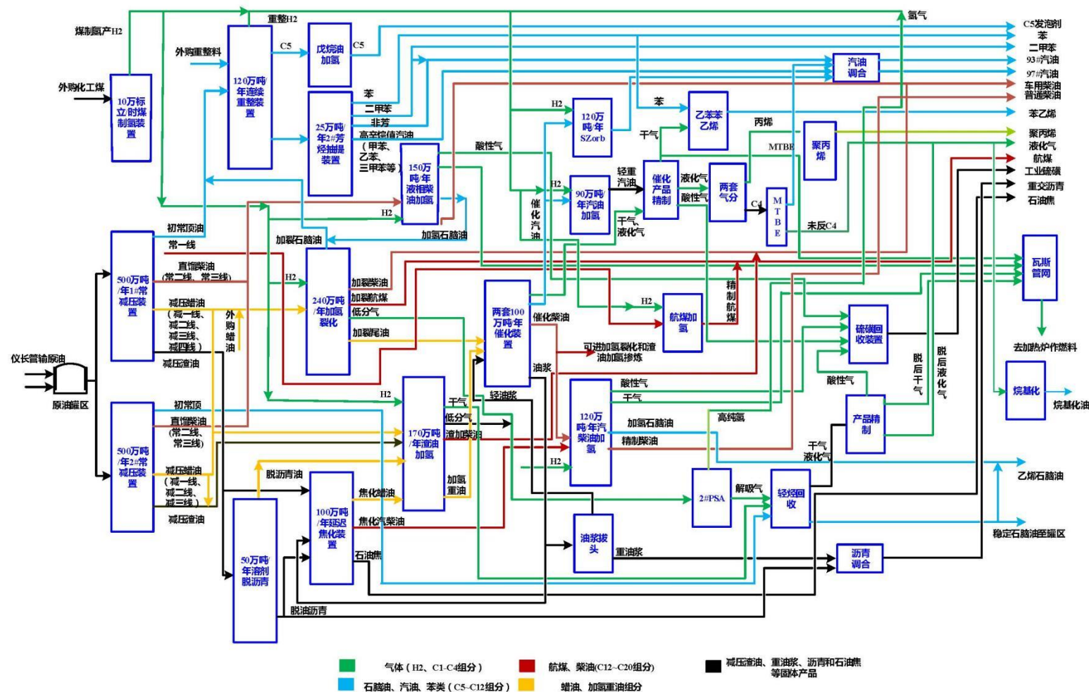
图1.1 九江石化2022年全厂加工总工艺流程图
